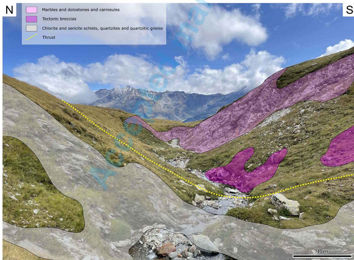
Fig. 36 - Geological scheme of Valle dei Buoi, 500 meters NNE from Lago Bianco.
